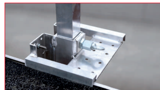
Bevestiging geklemd aan daktrim
