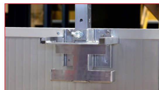
Bevestigingen geschroefd aan de voorzijde
