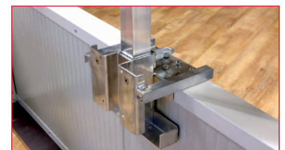
Bevestigingen geschroefd aan de bovenzijde
